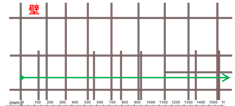
立面図（実際の配筋状況を作図）
